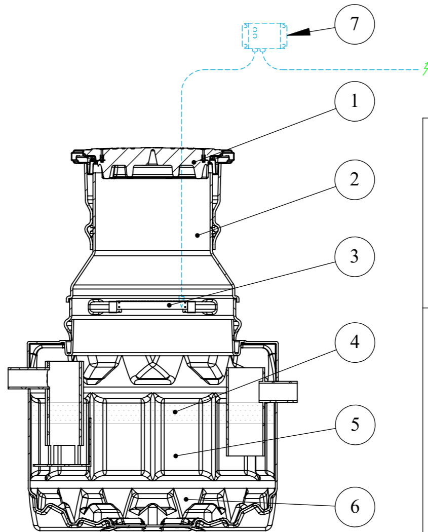
A-A
